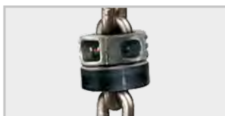
Prellgummi und Ketten- stopper aus Edelstahl am lastfreien Kettenende
